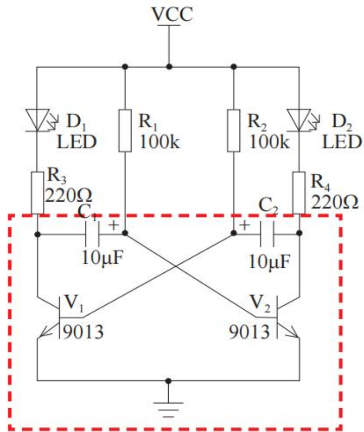
附图：多谐振荡器双闪灯电路
