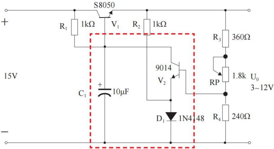
附图：可调式直流稳压电源
